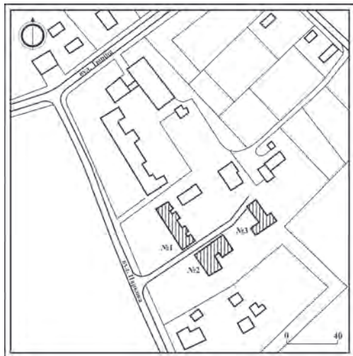
Село Олександропіль. Комплекс земської лікарні, поч. 1910-х рр. (схема розташування)
