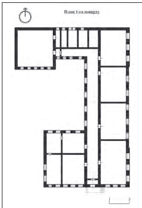
Село Широке. Будинок земської школи, поч. XX ст. (план будинку)
